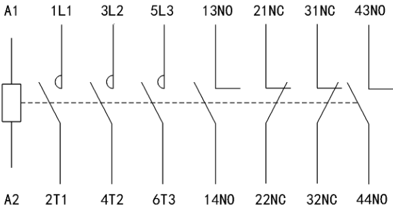
NDC5K-2400R/H 2700R/H 3200R/H 接线图
