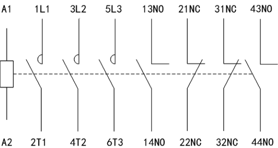
Wiring Diagram of NDC5K-2400R/H、2700R/H、3200R/H
