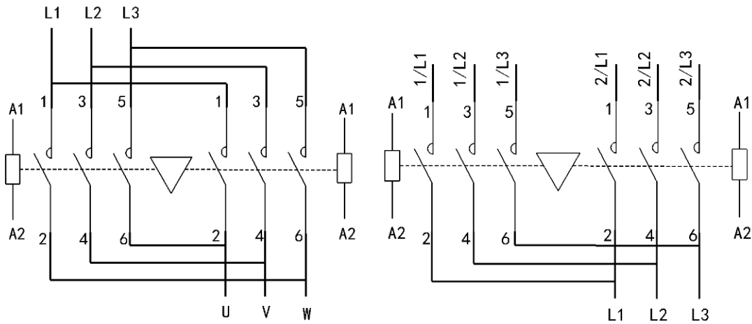
电动机控制可逆接触器接线图 配电用电源转换接线图 2) 主回路接线端子连接导线能力（见表 1）及力矩（见表 2）
